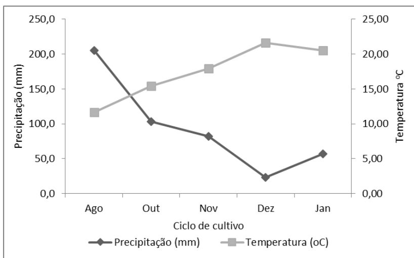
Figura 01. Dados referente a precipitação (mm) e temperatura (°C) durante o ciclo de cultivo. Quilombo, SC, Brasil. 2014.
