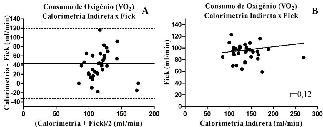
Figura 19 - Análise gráfica de Bland-Altman (A) e correlação de Pearson por regressão linear (B) do consumo de oxigênio ( \text{VO}_2 ) obtido por calorimetria ou por equação de Fick em cães anestesiados com isoflurano (1,4V%), sob ventilação mecânica e submetidos a estados hipo e hiperdinâmicos.
