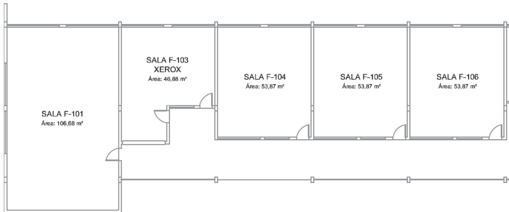
Planta Baixa Bloco F- Pavto Térreo
