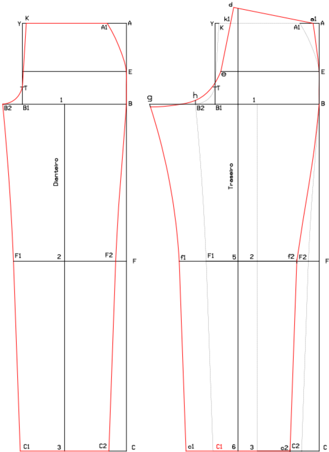
Diagrama 10 - Traçado básico da calça masculina
