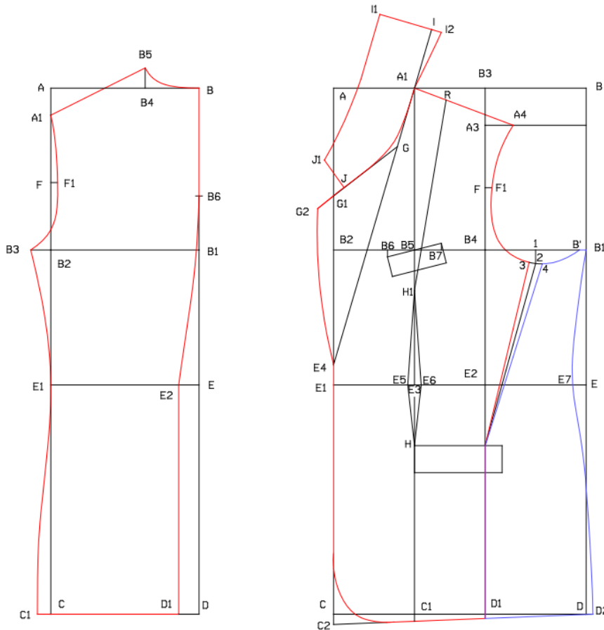
Diagrama 11 - Paletó masculino
