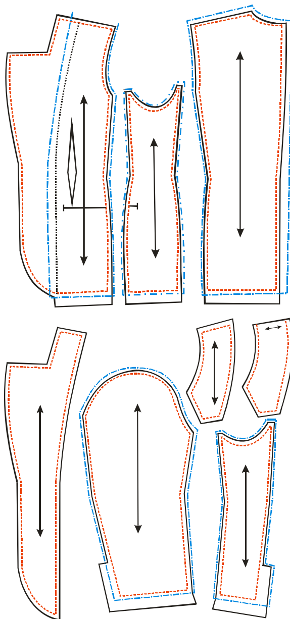
Figuras 38 – Forro do paletó
