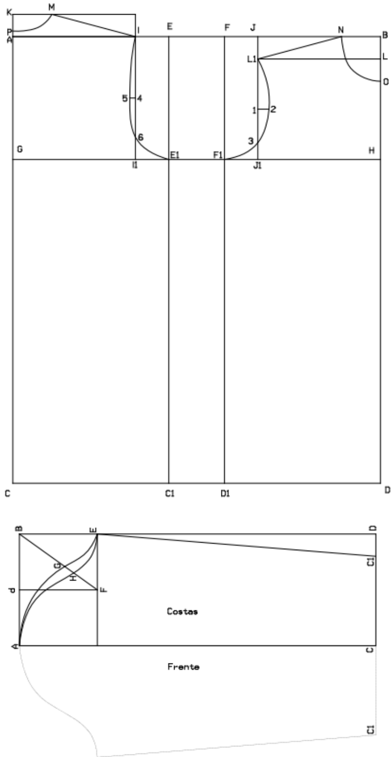
Diagrama 1 - Traçado Básico do corpo masculino
