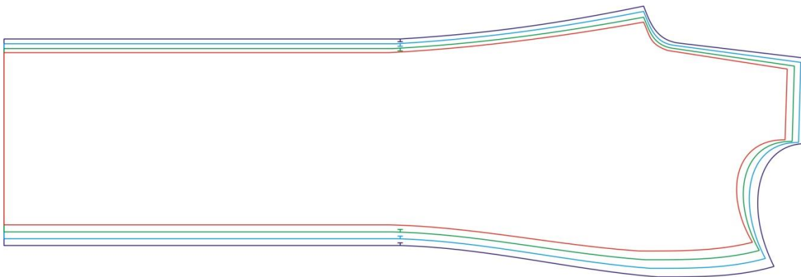
Figura 59 – Gradação do dianteiro
