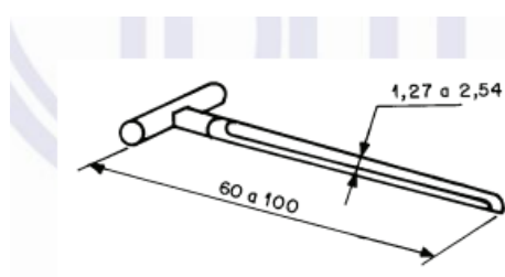
Figura B.3 – Amostrador “trier”
