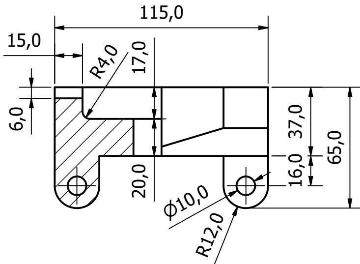
A-A ( 1 : 2 )
