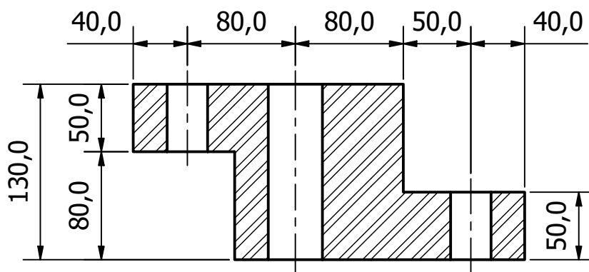
A-A ( 1 : 4 )
