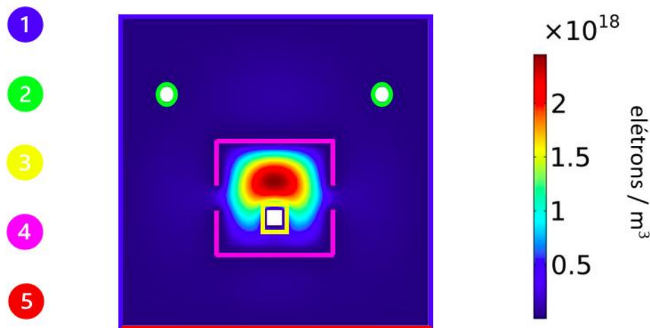
Figura 1. Densidade de plasma no modelo da gaiola catódica.
