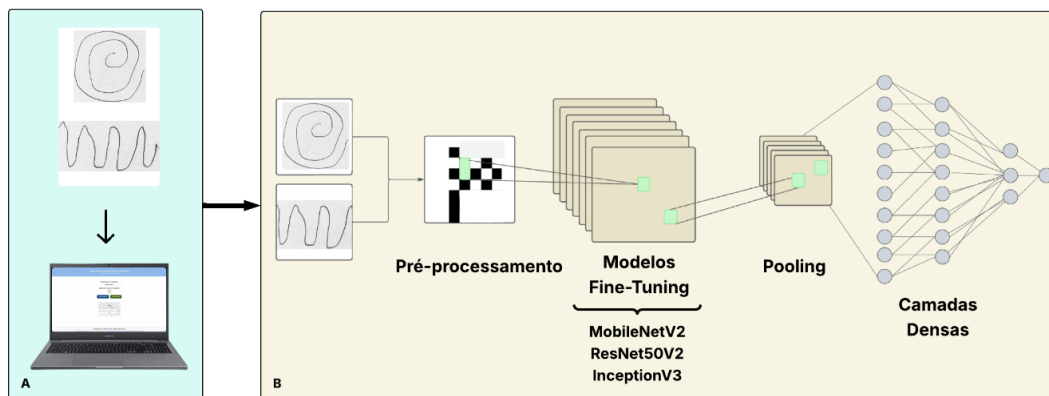
Figura 1: Ideia geral da construção dos modelos preditivos usando transfer learning . A) Representa os dois tipos do conjunto de dados, wave e spiral ; B) Processos de fine-tuning de redes neurais pré-treinadas.
